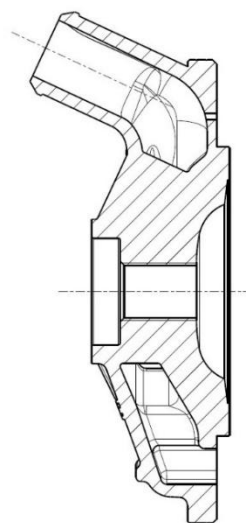
SEZIONE A-A
