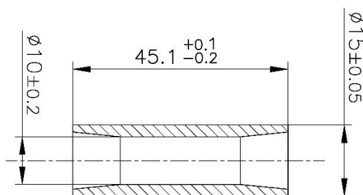
Axe de piston POIDS : 30g Min.
